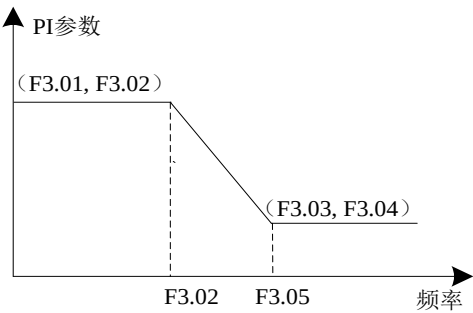
图 6-8 速度环 PI 参数示意图
