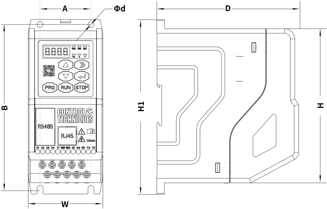
图 9-1 产品外形及安装尺寸
