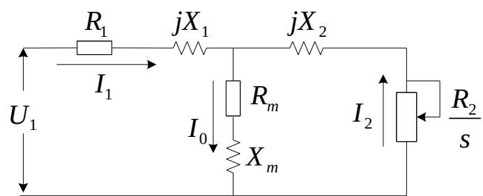
图 6-13 异步电机稳态等效电路图
