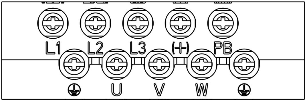
图 3-3 Captain XL 系列带制动单元的主回路端子配线图
