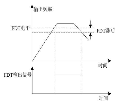
图 6-22 FDT 电平示意图
