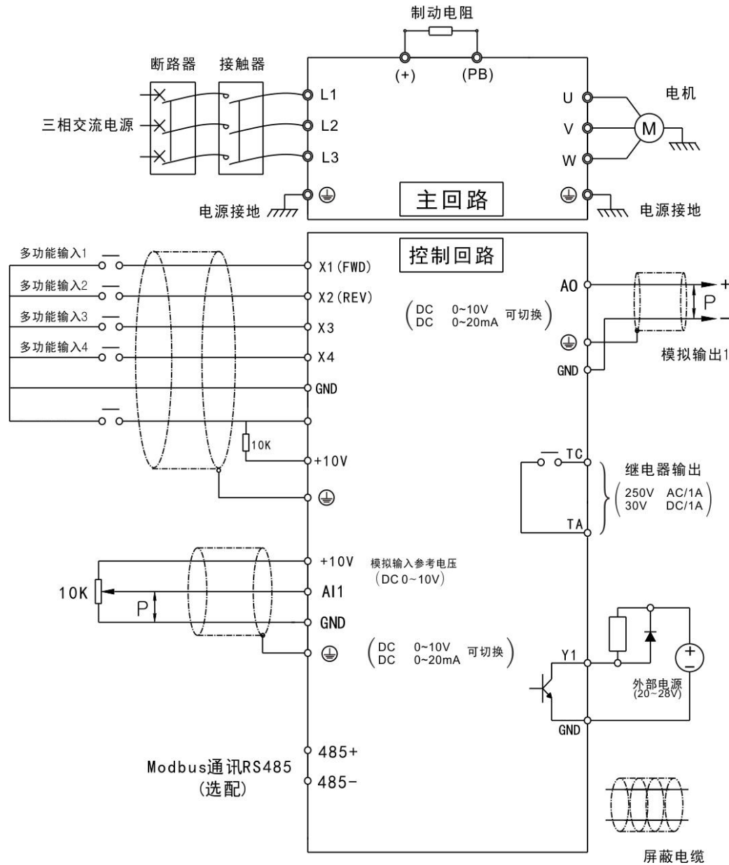
图 3-2 Captain XL 系列基本配线图
