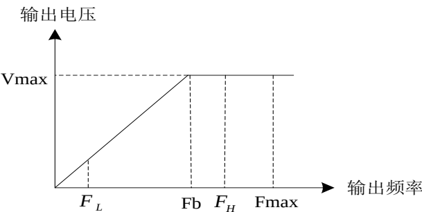
图 6-1 输出频率与输出电压关系图
