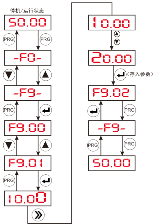
图 4-2 三级菜单操作流程图
