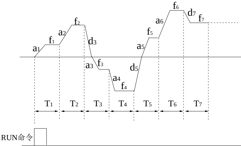
图 6-26 PLC 运行示意图
