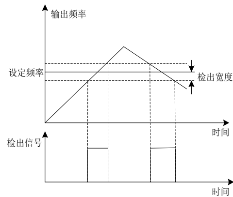
图 6-21 频率到达检出宽度示意图
