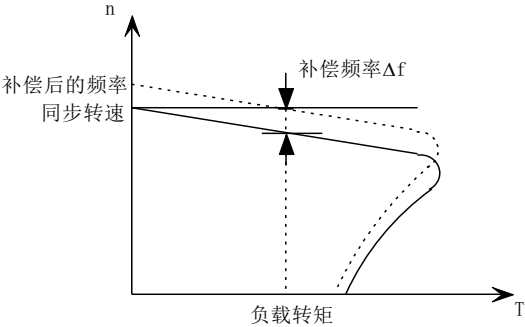
图 6-12 自动转差补偿
