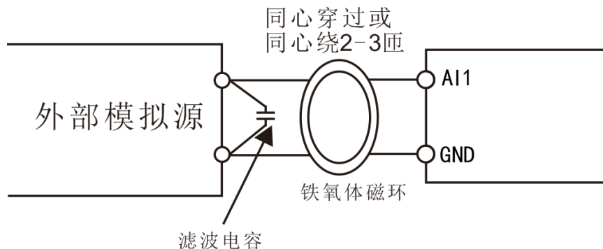
图 3-5 模拟输入端增加滤波器接线示意图
