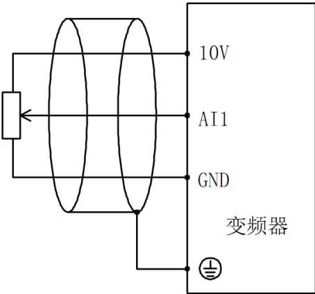
屏蔽线近端接地
