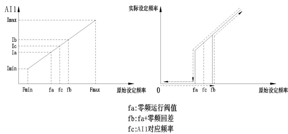
图 6-7 零频回差运行
