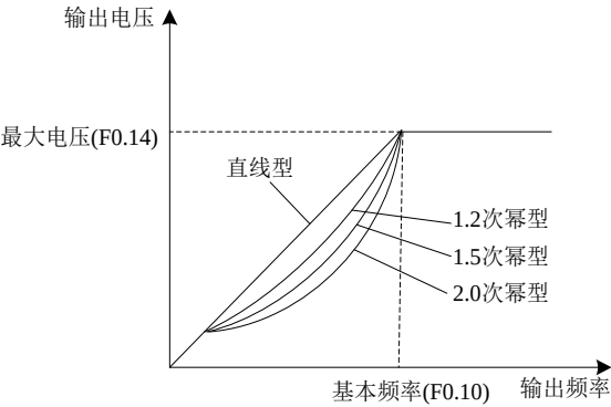
6-9 V/F 曲线示意图
