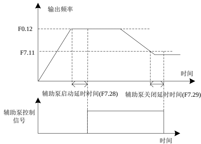
图 6-23 恒压供水辅助泵控制信号
